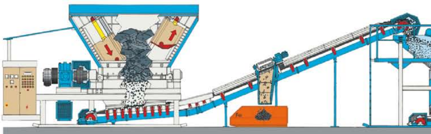
Schematische Darstellung des Materialflusses
